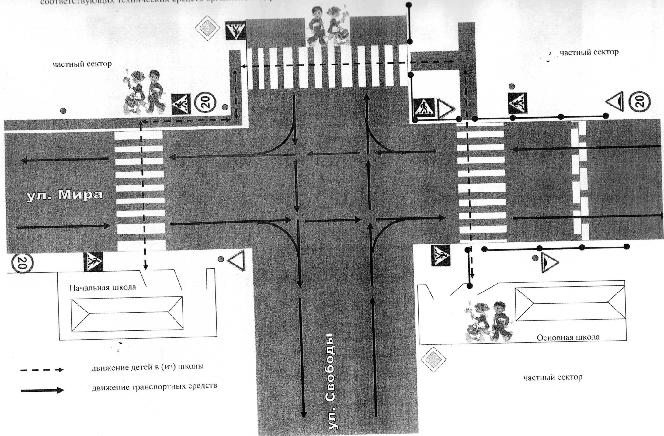
Схема №2. Организация дорожного движения в непосредственной близости от образовательных учреждений, маршруты движения детей и расположение парковочных мест соответствующих технических средств организации дорожного движения, маршруты движения детей и расположение парковочных мест.
