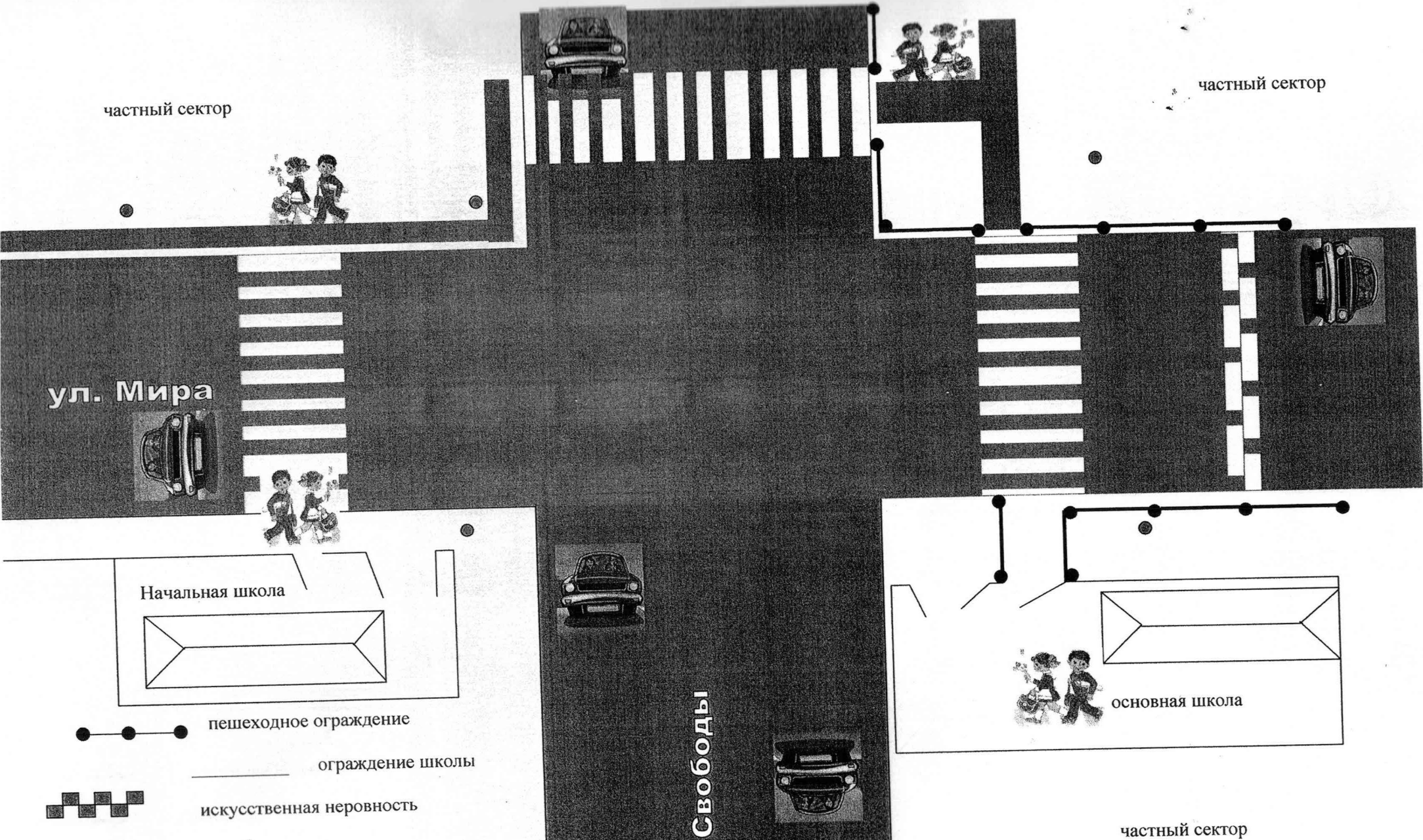
Схема №1. Район расположения образовательной организации, пути движения транспортных средств и детей (обучающихся).
